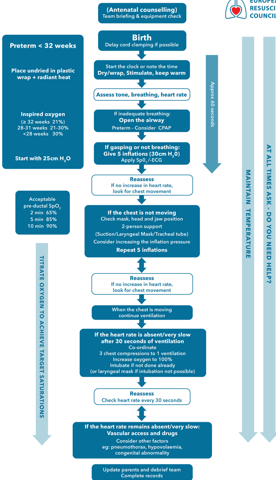
Fig. 14 - NLS algorithm.
